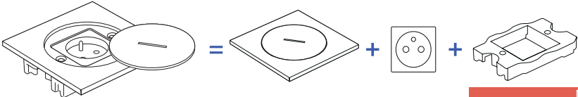
Couvercle à ouverture standard + mécanisme + support mécanisme
