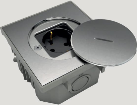
PRISE SCHUKO - BFC101/2
